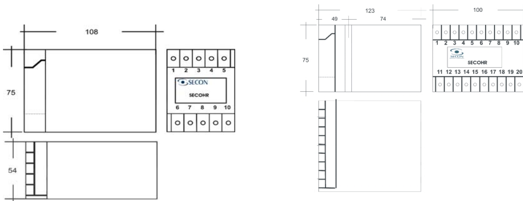
Encapsulamento Tipo1
