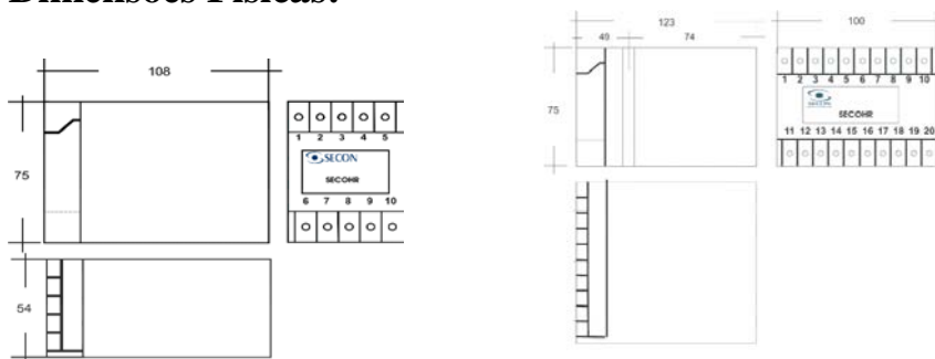
Encapsulamento Tipo1
