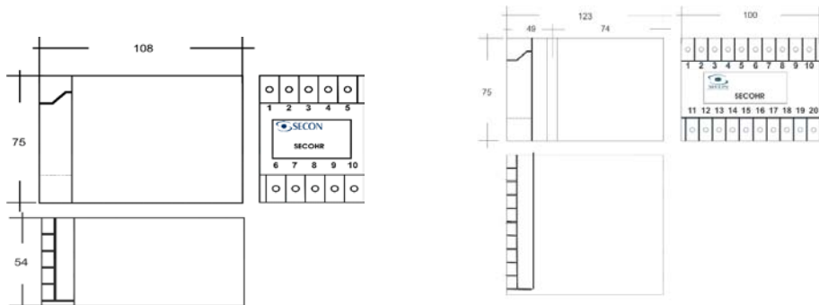
Encapsulamento Tipo1
