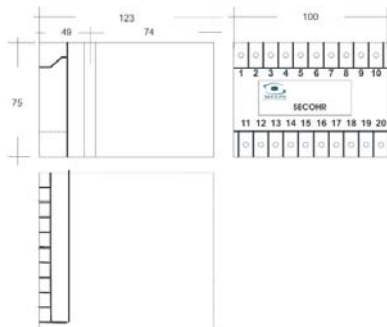
Encapsulamento Tipo2
