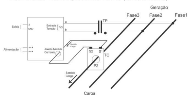
Medida Trifásica - Sistema Equilibrado com TC e TP (1 elementos, 3 fios)
