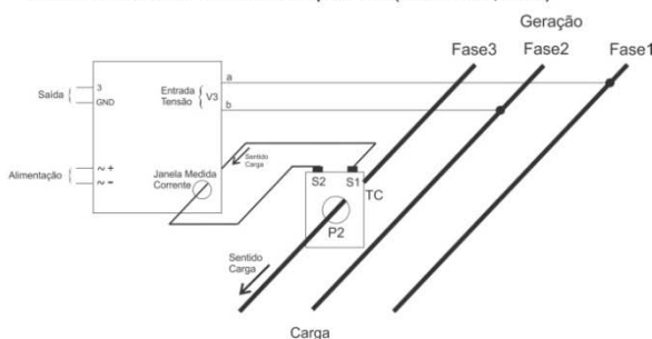
Medida Trifásica com TC - Sistema Equilibrado (1 elementos, 3 fios)
