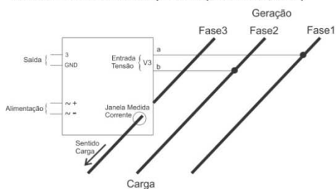
Medida Trifásica - Sistema Equilibrado (1 elementos, 3 fios)
