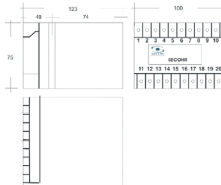
Encapsulamento tipo 2
