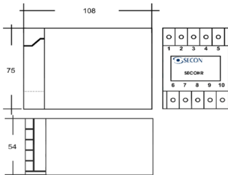
Encapsulamento tipo 1
