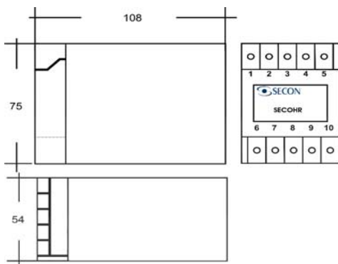
Encapsulamento Tipo1
