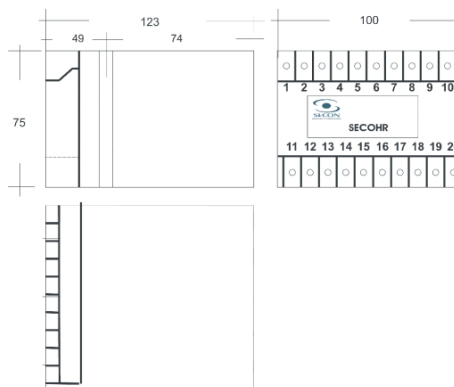
Encapsulamento Tipo2
