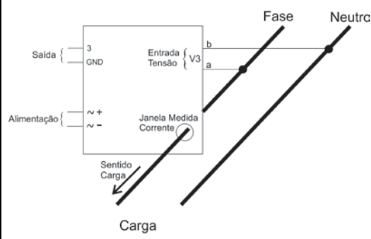
Medida F-N (1 elementos, 2 fios)
