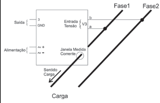
Medida F-F (1 elementos, 2 fios) 120° ou em quadratura (90°)
