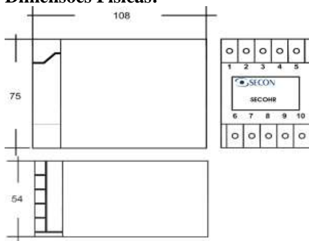
Encapsulamento Tipo1
